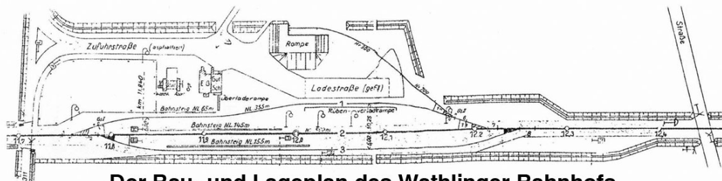
Der Bau- und Lageplan des Wathlinger Bahnhofs
